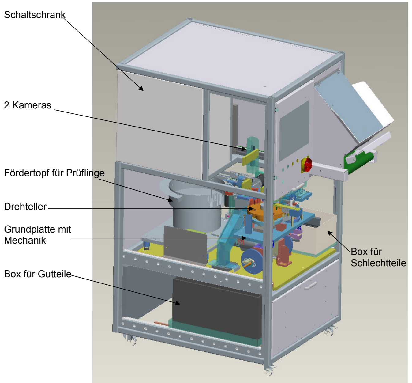
Bild2: Gesamtanlage ohne Verkleidung
